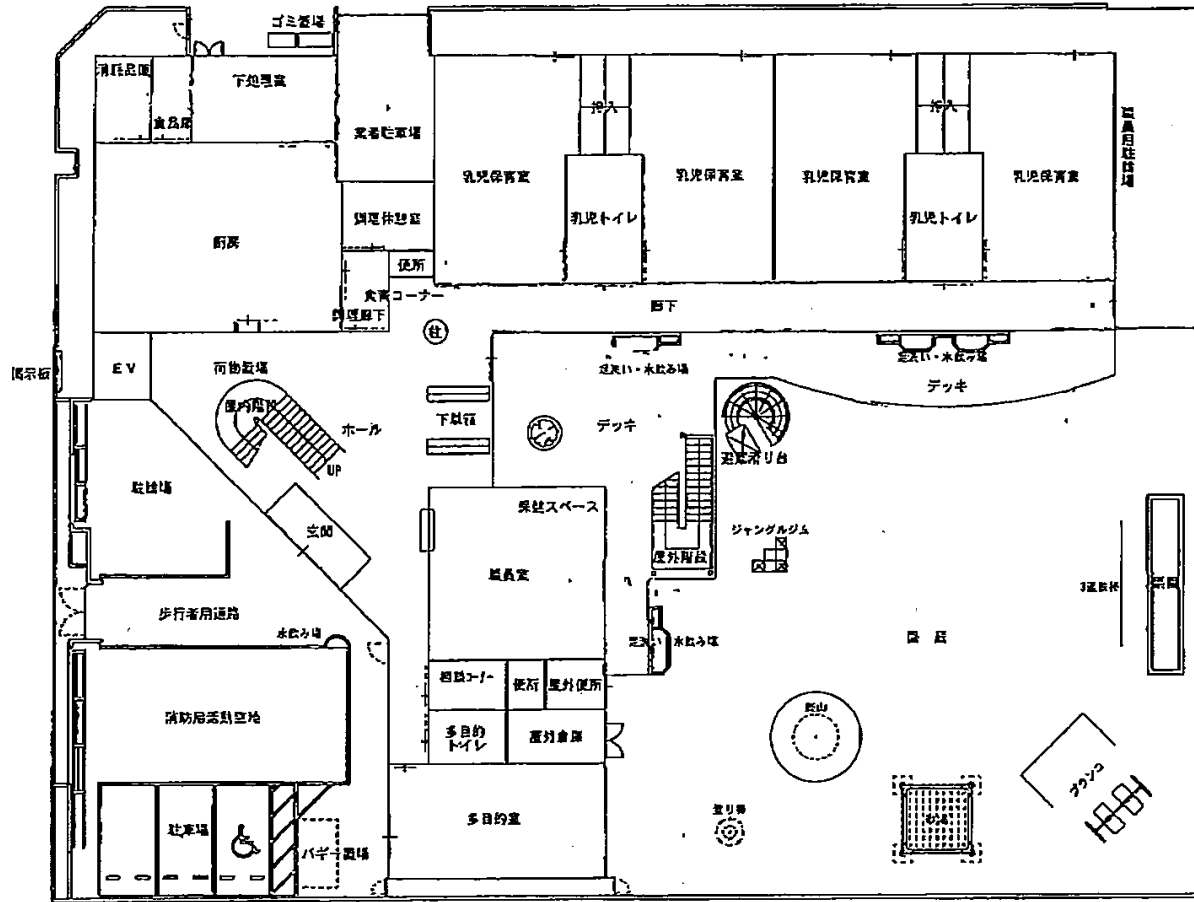
《 1階平面図 》
