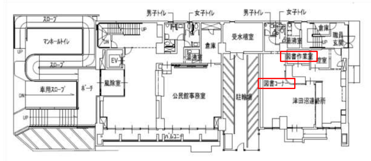
東部公民館等複合施設 1 階平面図（改修後）
