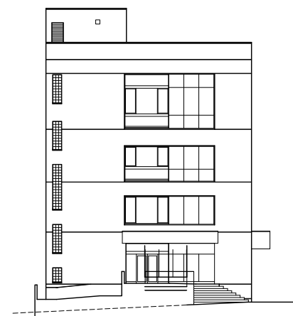
西側立面图
