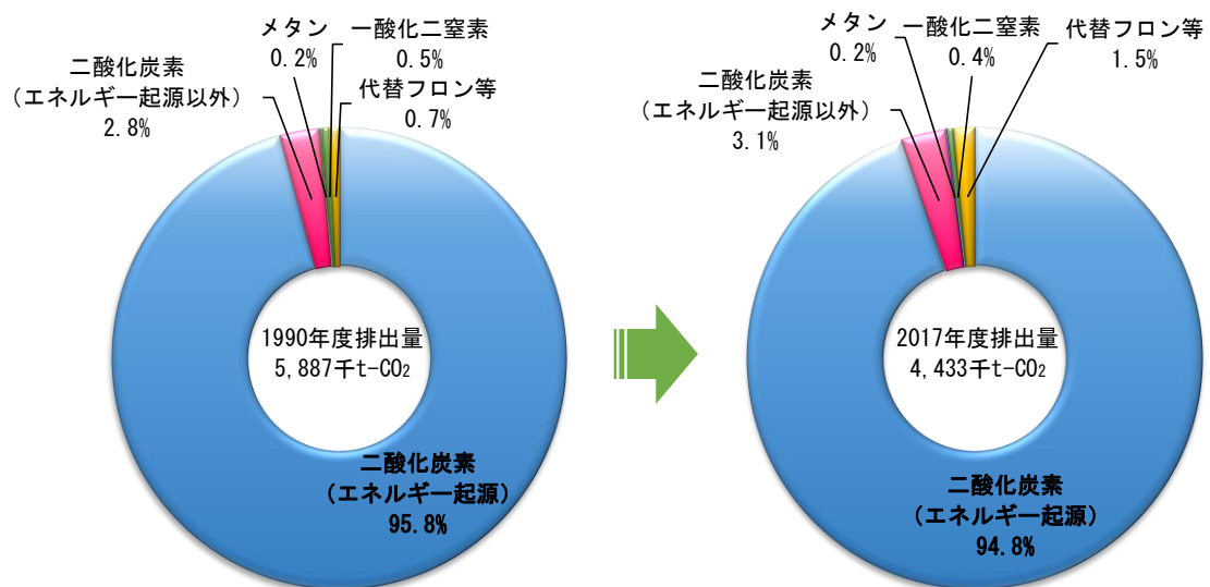
図 V-12 温室効果ガス別排出割合の変化 (左：1990 年度（平成 2 年度）、右：2017 年度（平成 29 年度）)
