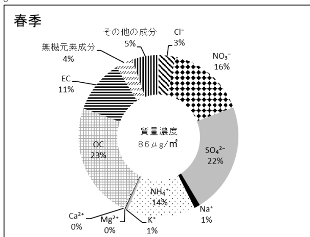
図2-1-36 PM2.5の成分組成内訳 (春季 R4.5.12~5.26 高根台局)
