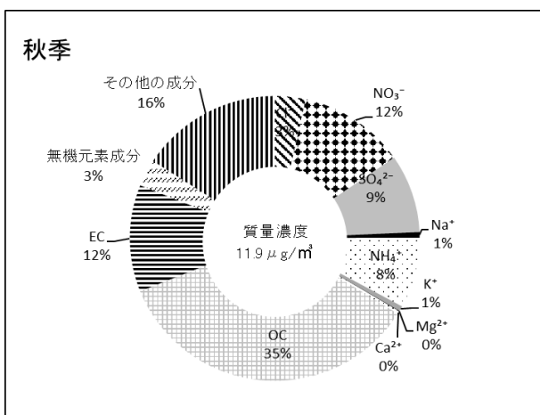
図2-1-38 PM2.5の成分組成内訳 (秋季 R4.10.20~11.3 高根台局)
