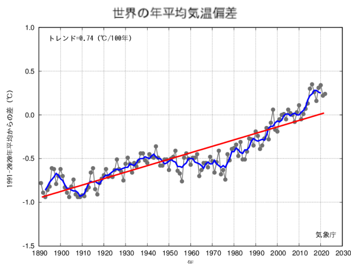
図 2-4-1 世界の年平均気温の経年変化 (1891～2022 年) 出典: 気象庁
