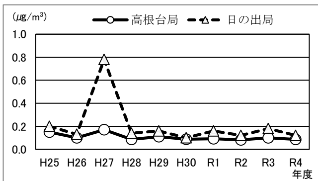
図 2-1-31 1,3-ブタジエンの経年変化 (指針値: 2.5μg/m³)
