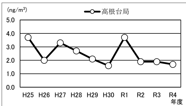
図 2-1-29 ニッケルの経年変化 (指針値: 25ng/m³)
