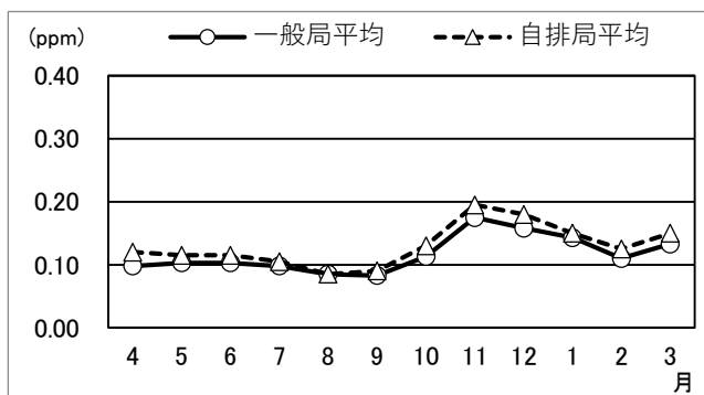
図 2-1-17 非メタン炭化水素(3 時間値)の経月変化
