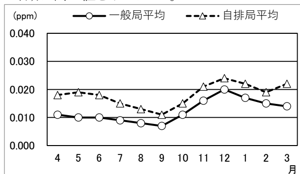
図 2-1-15 二酸化窒素の経月変化
