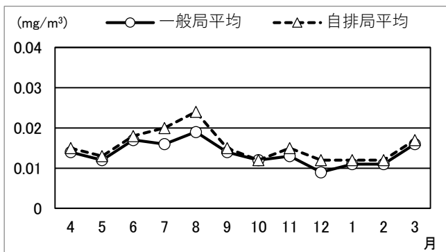
図 2-1-9 浮遊粒子状物質の経月変化
