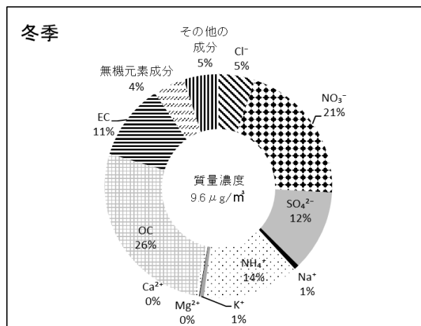
図2-1-39 PM2.5の成分組成内訳 (冬季 R5.1.19~2.2 高根台局)
