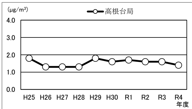
図 2-1-33 塩化メチルの経年変化 (指針値: 94μg/m³)
