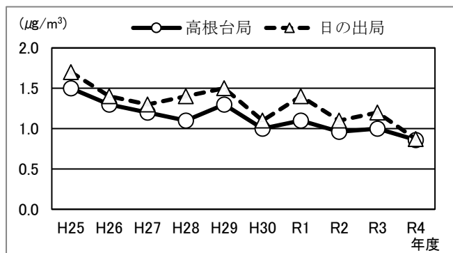
図2-1-20 ベンゼンの経年変化 (環境基準値: 3μg/m³)
