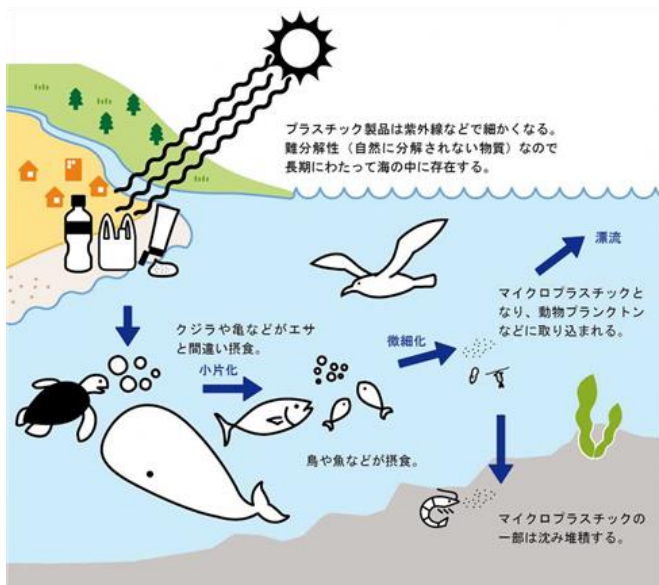
マイクロプラスチックができる仕組み
