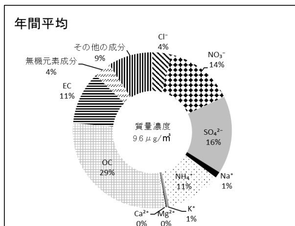
図2-1-35 PM2.5の成分組成内訳(年間平均:高根台局)
