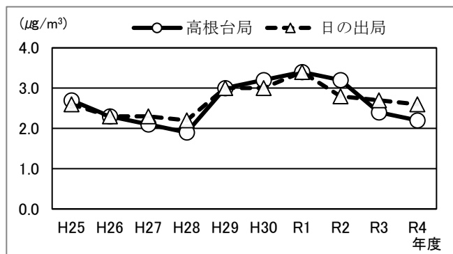
図 2-1-34 アセトアルデヒドの経年変化 (指針値: 120μg/m³)
