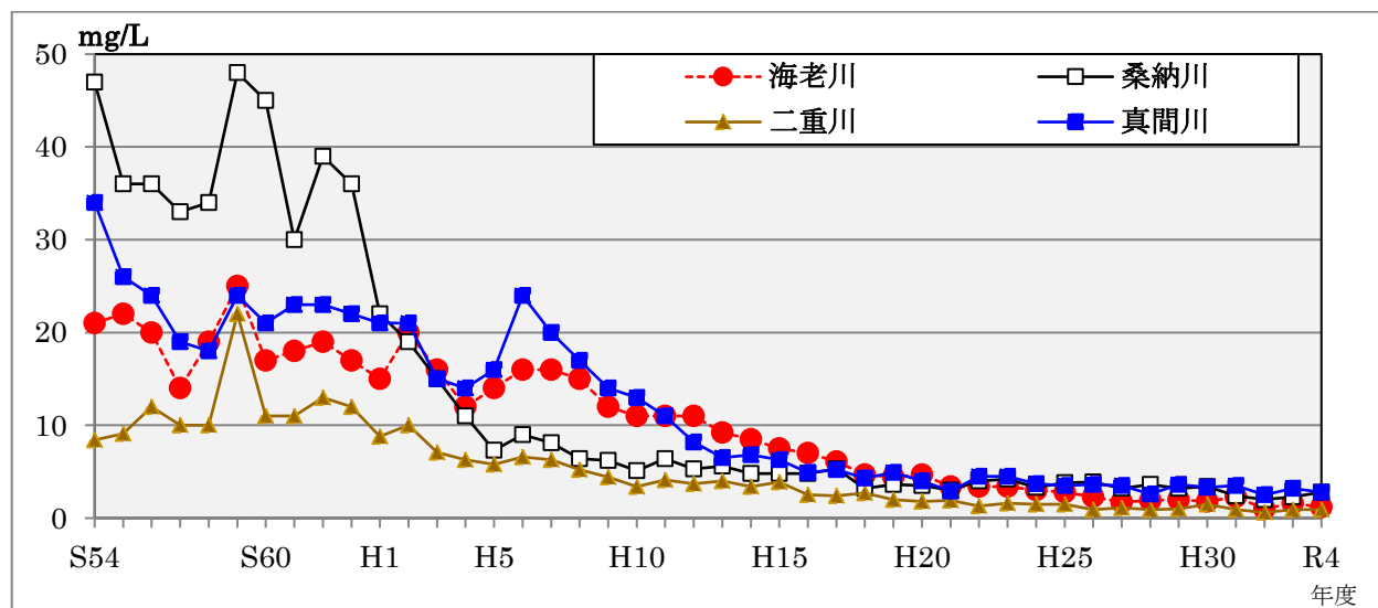
図 2-1-42 河川の BOD 経年変化(年平均値)
