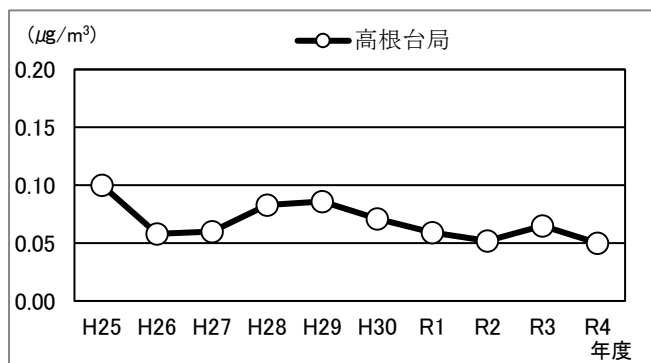
図2-1-22 テトラクロロエチレンの経年変化 (環境基準値: 200μg/m³)
