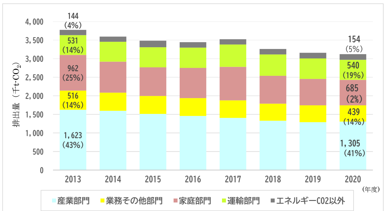
図 2-4-4 船橋市における部門別二酸化炭素排出量の内訳
