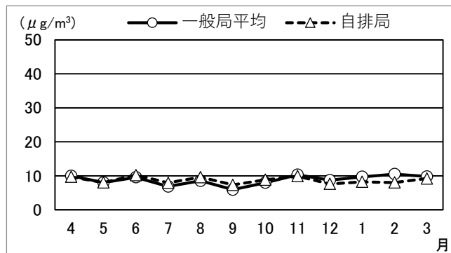
図 2-1-11 微小粒子状物質の経月変化
