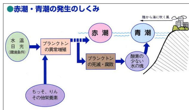
図 2-2-9 赤潮・青潮の発生の仕組み
