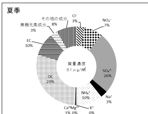
図2-1-37 PM2.5の成分組成内訳 (夏季 R4.7.21~8.4 高根台局)
