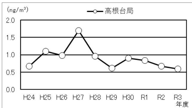
図 2-1-30 砒素の経年変化 (指針値: 6ng/m³)
