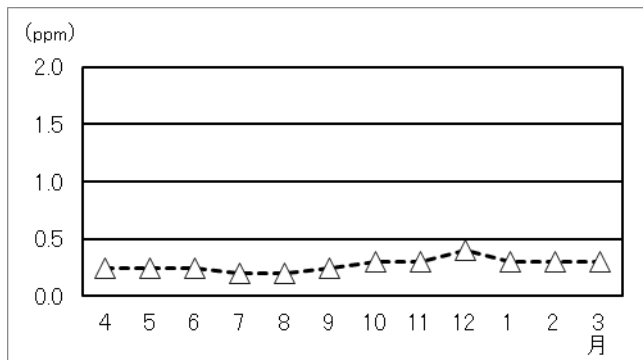
図 2-1-19 一酸化炭素の経月変化(自排局平均)
