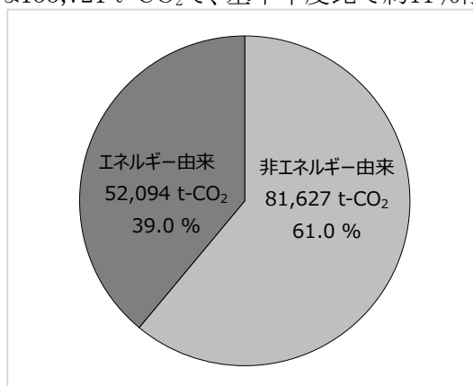
図 2-4-7 温室効果ガス由来別排出量(市事業全体)
