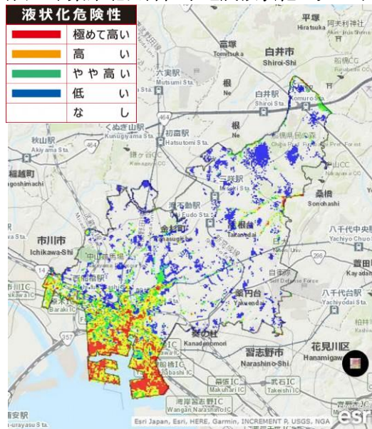
図表 千葉県北西部直下地震液状化の発生予想
