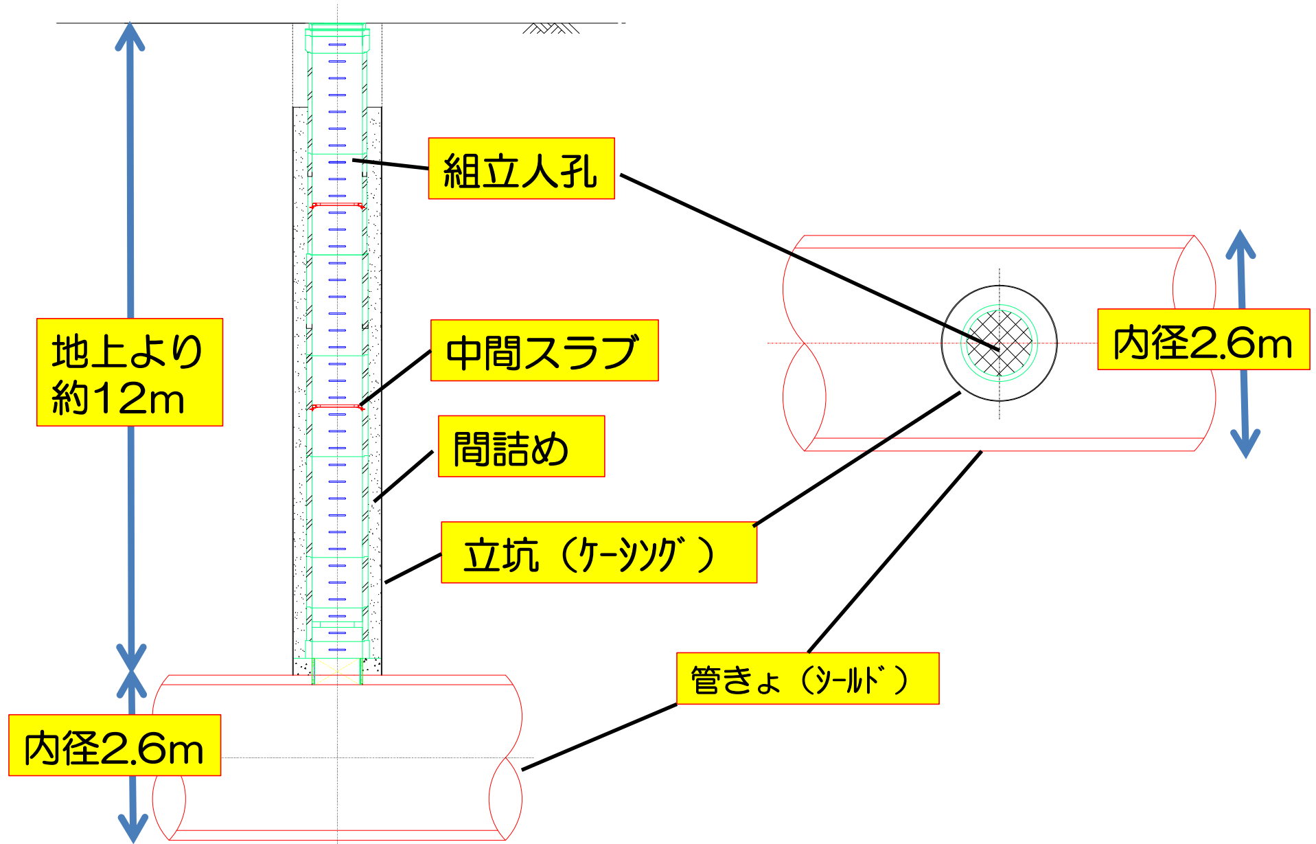
断面図
