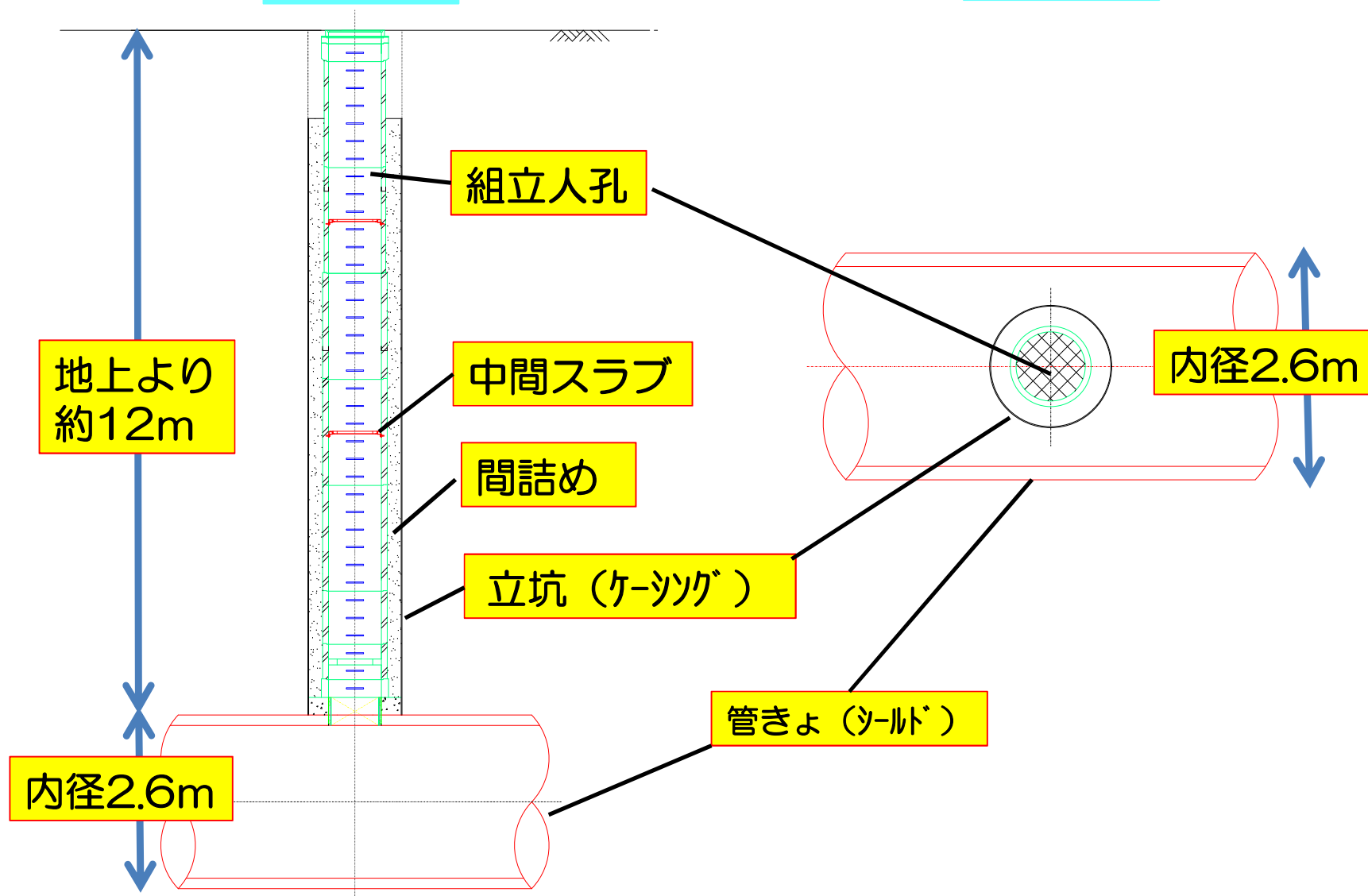
断面図
