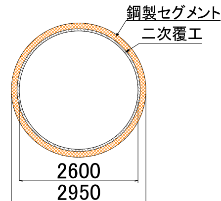
鋼製セグメント区間
