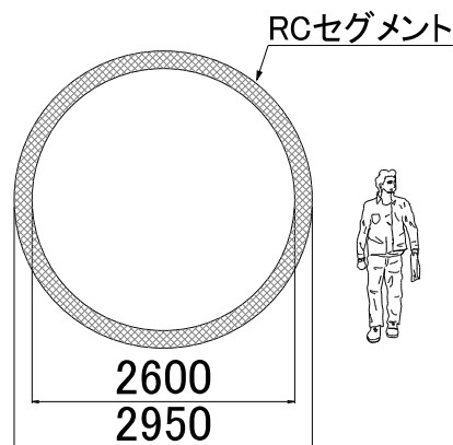
RCセグメント区間
