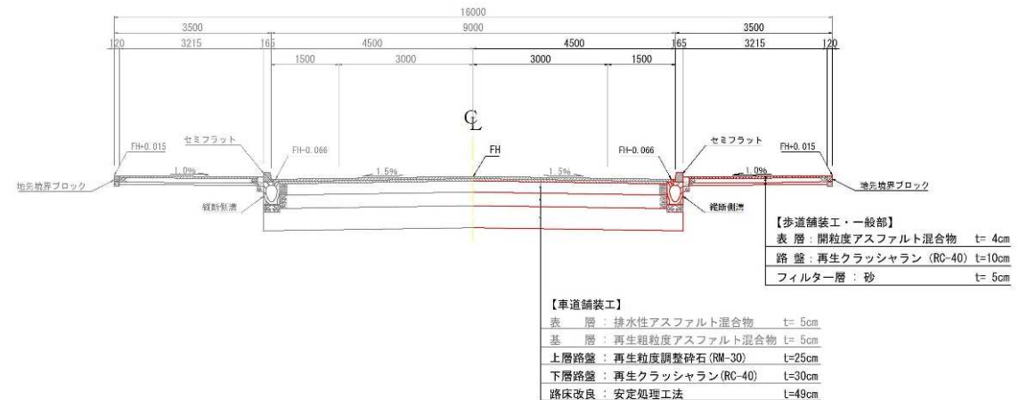
標準断面図
