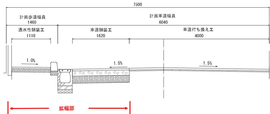
標準断面図
