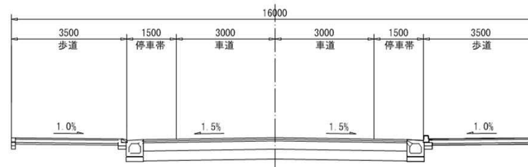
標準断面図
