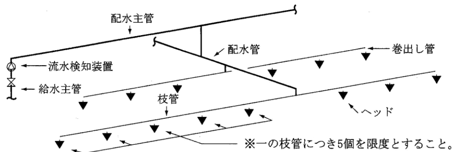
第6-17図 [配管の名称及び枝管とヘッドの取付け例]
