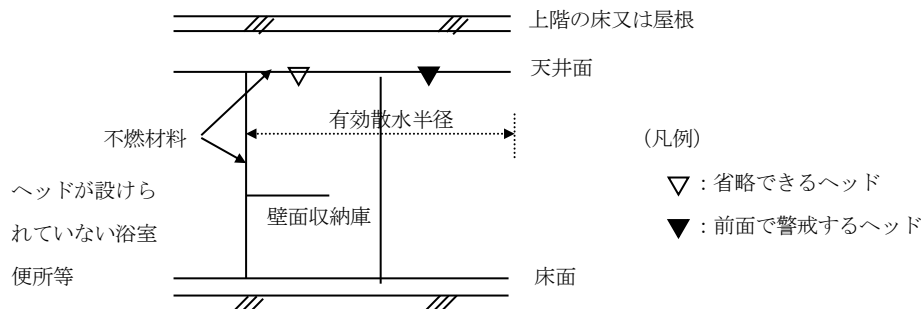
第6-3図 壁面収納庫の上部のヘッドを省略した例
