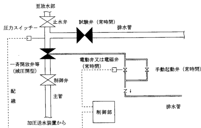
図5 減圧方式の一斉開放弁等の廻りの配管図例
