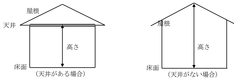
第6-21図 〔床面から天井までの高さの例〕
