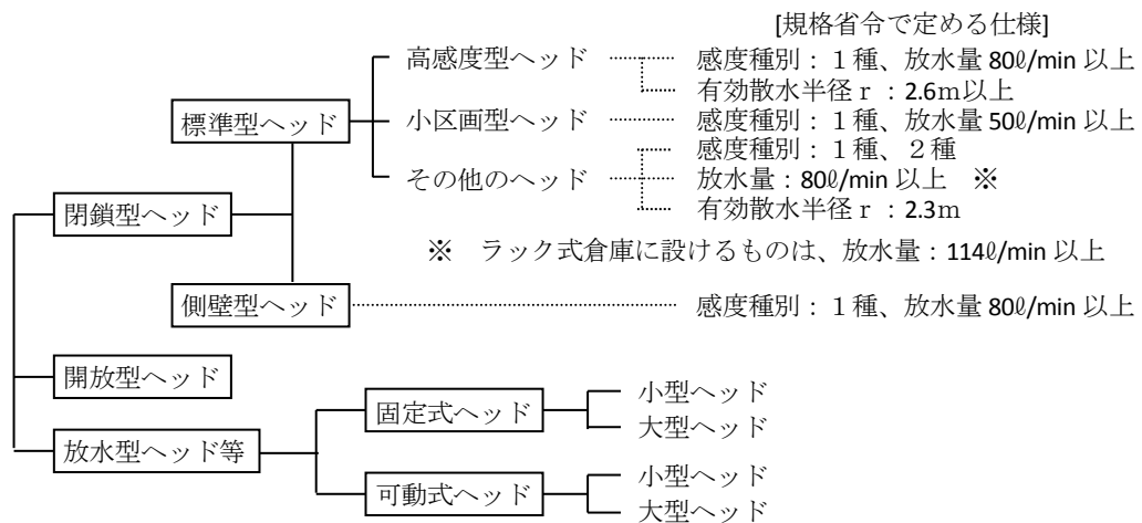
第6-1図 [スプリンクラーヘッドの体系]
