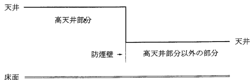
図3 防煙壁等の設置例
