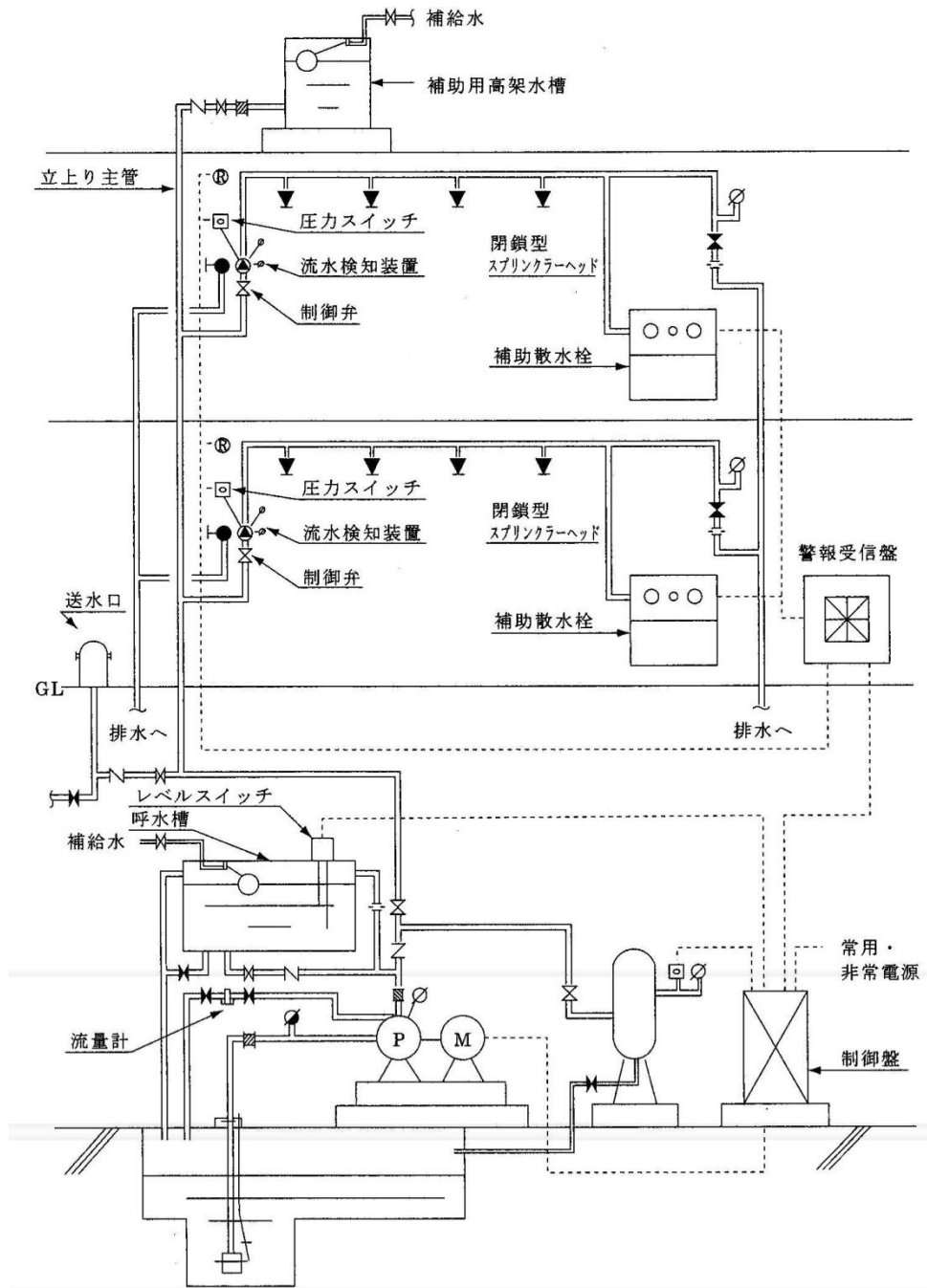
別図第6-1 閉鎖型スプリンクラー設備の配管系統別例
