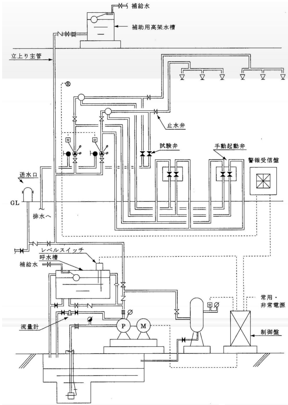
別図第6-2 開放型スプリンクラー設備の配管系統別例
