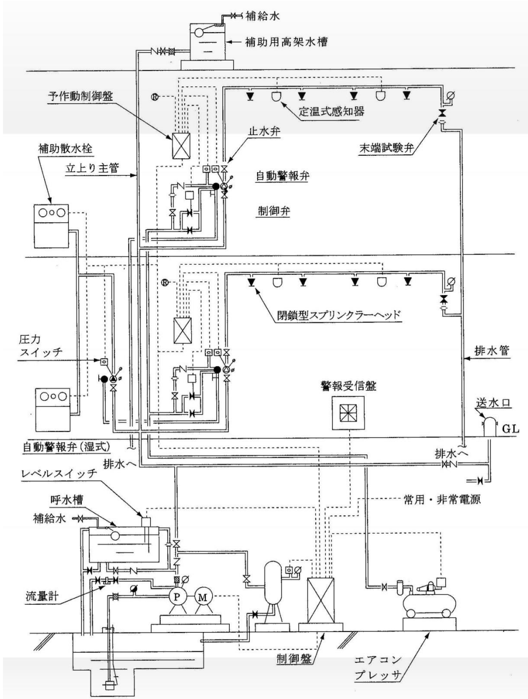
別図第6-3 予作動式スプリンクラー設備の配管系統別例
