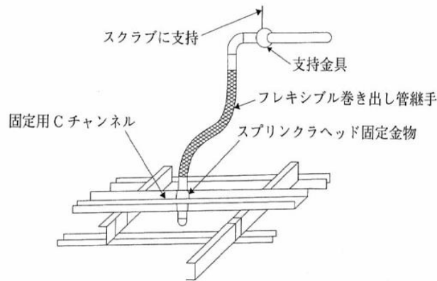
スプリンクラーヘッド等の耐震措置例
