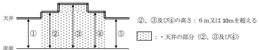
第6-22図 〔同一の空間の高天井部分(②, ③及び④)としての部分の例〕
