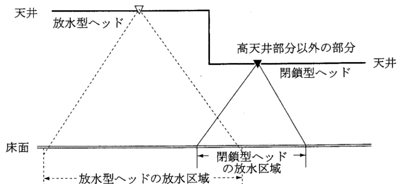
図4 放水区域等が相互に重複する設置例
