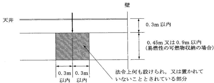
第6-13図 [標準型ヘッド（小区画型ヘッドを除く。）：断面]
