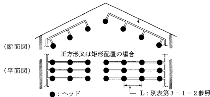
第6-11図 正方形又は矩形配置の場合の例
