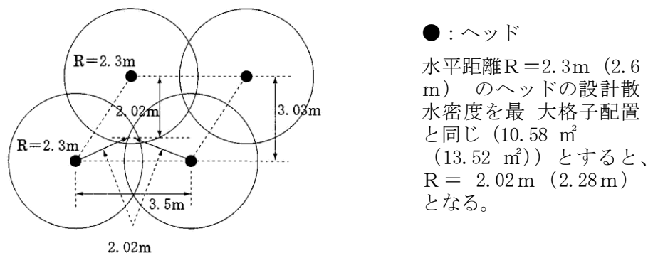
第6-10図 散水密度が低下しないようにした千鳥型配置の例
