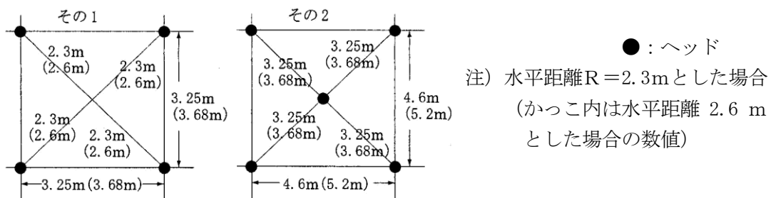
第6-9図 格子配列の例
