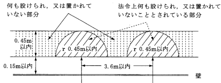
第6-15図 [側壁画ヘッドの場合：平面]
