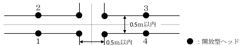
第6-19図 放水区域の重複例 ◎：開放型ヘッド
