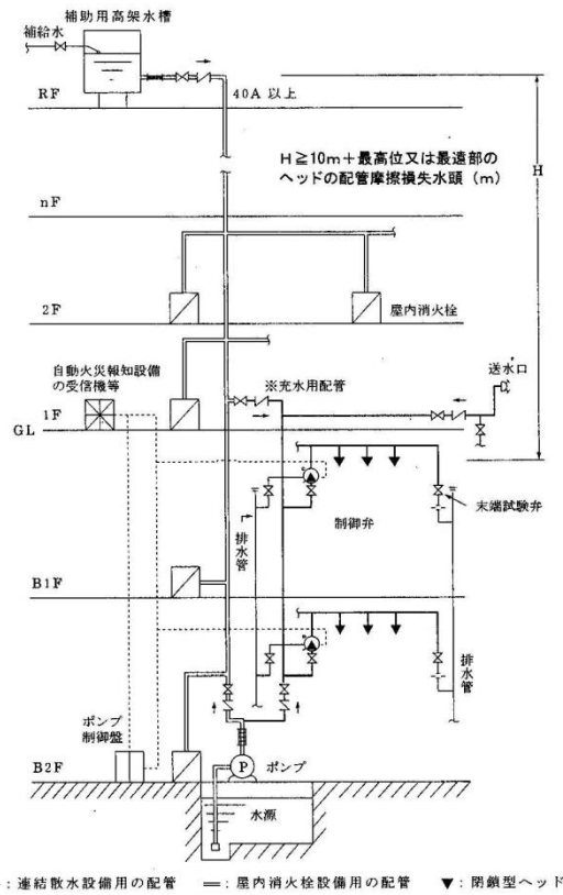
別図第 22-3 屋内消火栓設備兼用方式の配管系統例
