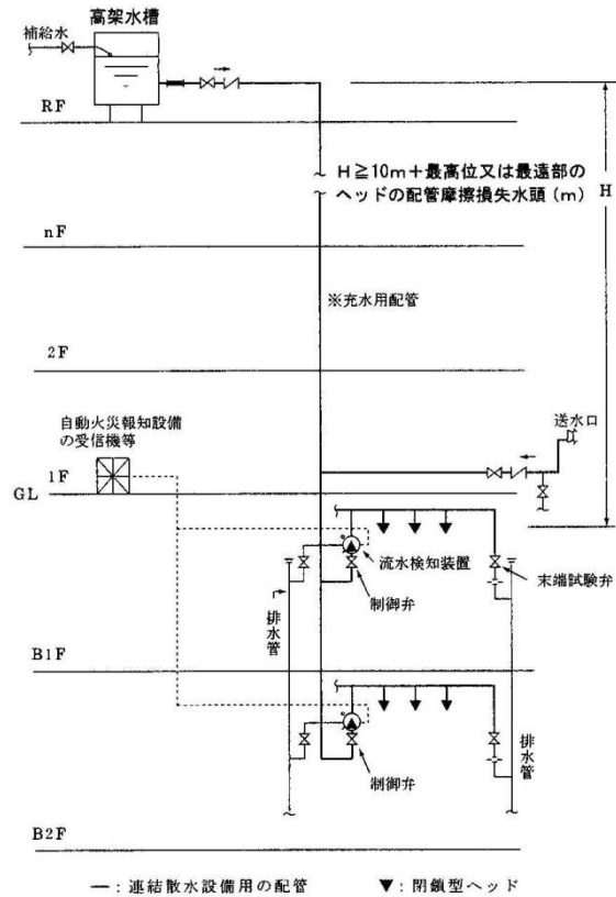
別図第 22 - 5 配管充水方式の配管系統例
