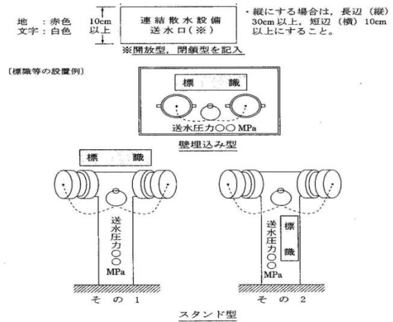
別図第 22-2 連結散水設備の送水口の標識等
