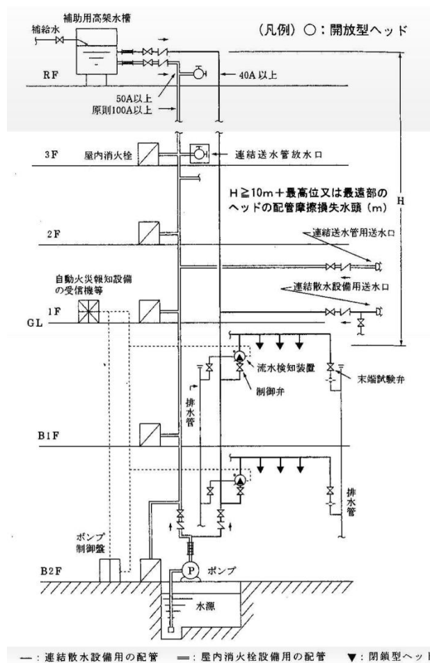
別図第 22-4 屋内消火栓設備兼用方式の配管と連結送水管の主管を兼用した場合の系統例
