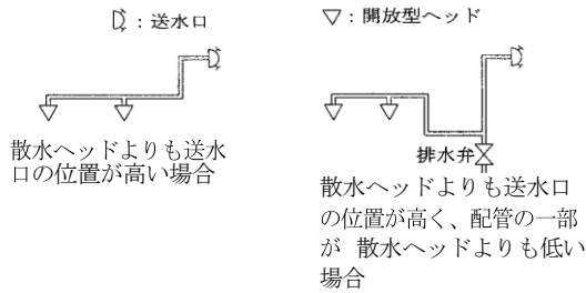
別図第 22-1 排水弁の設置 (例)
