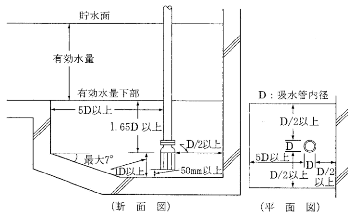
第4-5図 サクションピットを設ける場合の例
