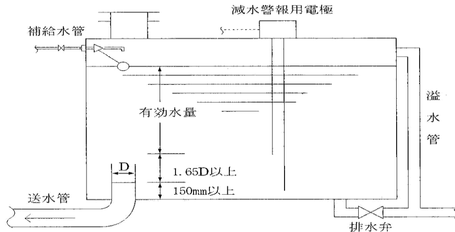
[低面より取出す場合の例] 注) D：送水管内径 第4-9図 他の水槽と併用する場合の有効水量
