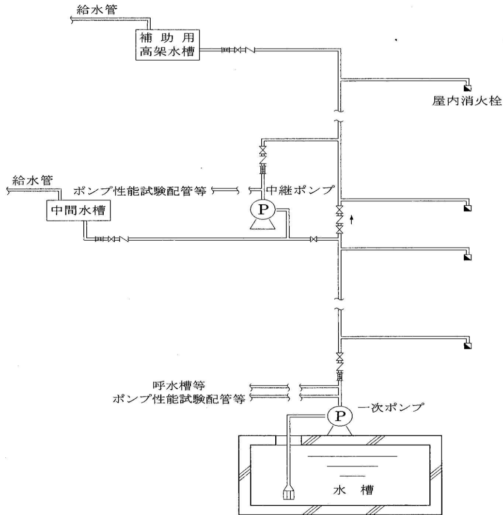
第4-4図 中継ポンプを設ける方法の例
