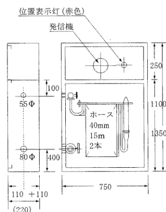
1号消火栓用箱内部の構造例 第4-13図
