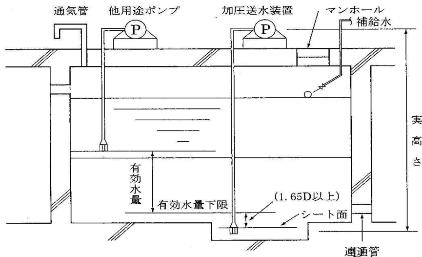
第4-8図 他の水槽と併用する場合の有効水量
