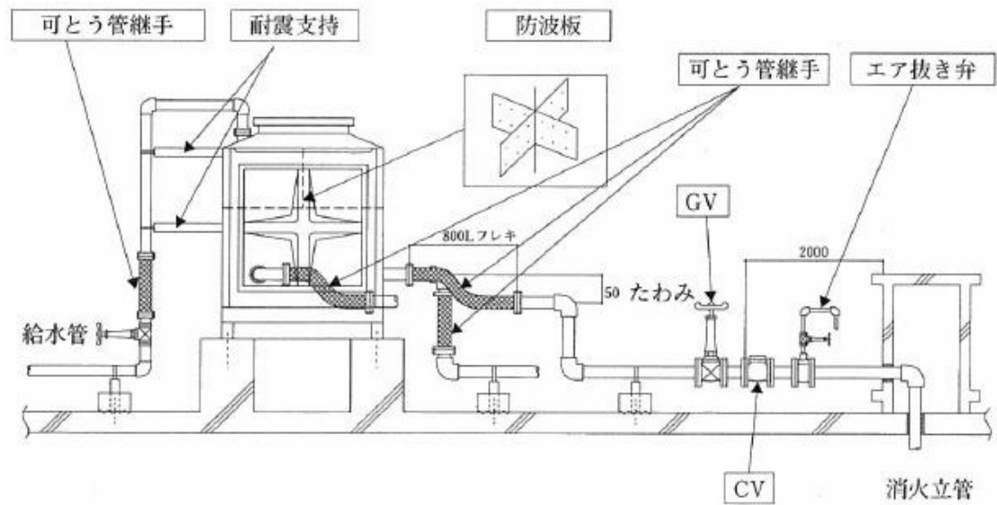
消火用水槽の耐震措置例
