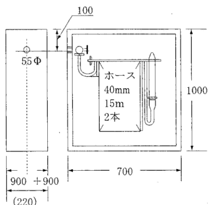
1号消火栓用箱内部の構造例 第4-13図
