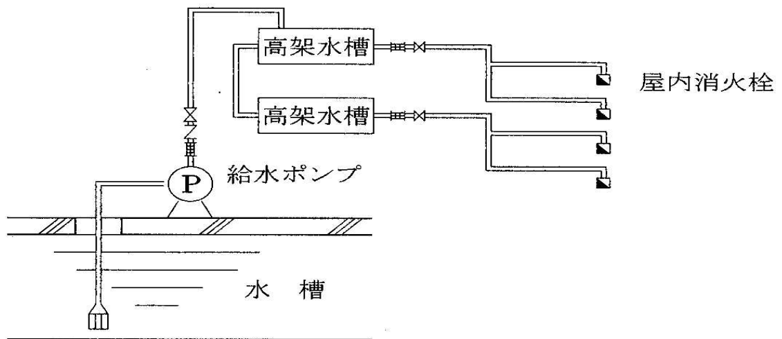
第4-2図 高架水槽の設置高さを考慮して設ける方法の例
