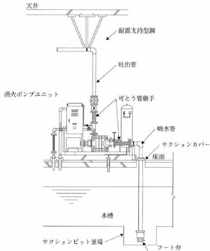
ポンプユニット耐震措置例 第4-12図
