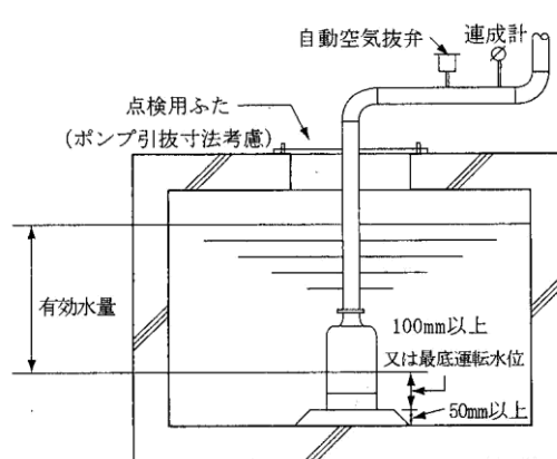
[サクションピットを設けない場合の例]
