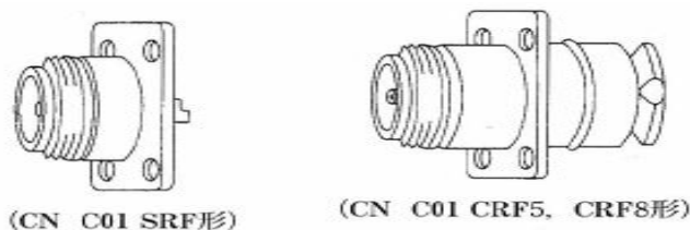
第 25—1 図 JIS C 5411 C01 形コネクタ外観図
