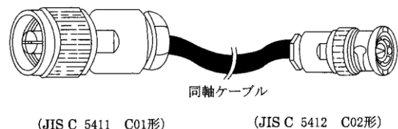
別図第 25-3 接続用の同軸ケーブル外観図
