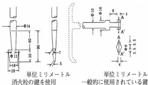
別図第 25-2 鍵の形状
