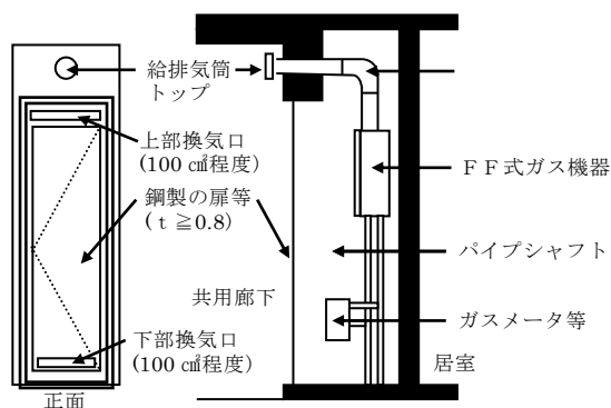
第 12－2 図 FF式ガス機器のパイプシャフト内設置の例
