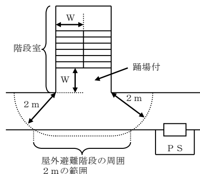
(屋外避難階段の例)
