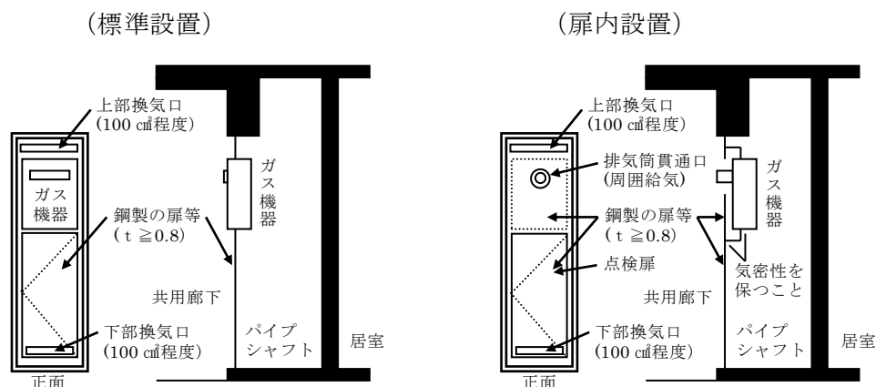
第12-1図 標準設置と扉内設置の例
