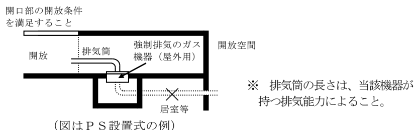
第 12－8 図 開口部位置の特例の例
