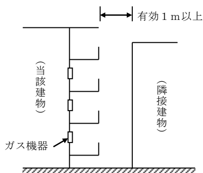
第 12-11 図参照 隣接建物との離隔距離の例
