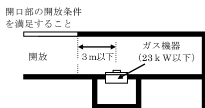
第 12－9 図 開口部位置の特例の例
