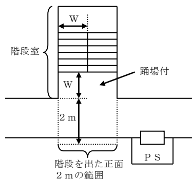
(屋外階段の例)
