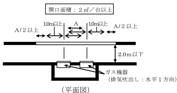
第 12-7 図 前面開口部条件の例
