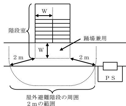
(屋外避難階段の例)
