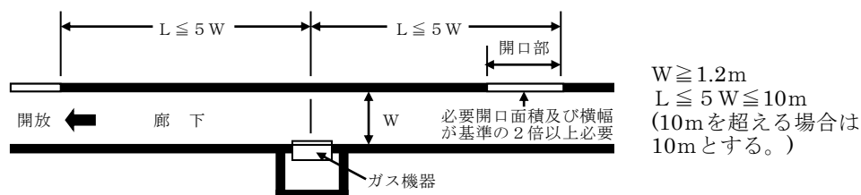
第 12-5 図 開口部の範囲の例
