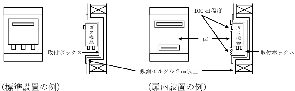
第 12－14 図 壁組込設置式の例
