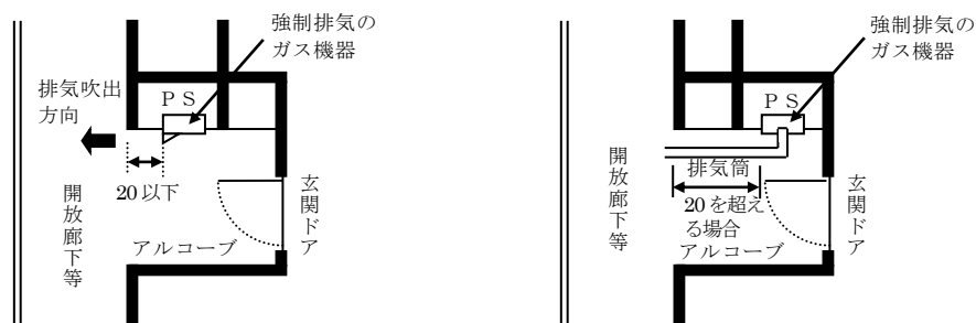
第 12-10 図 アルコーブへの設置の例（単位 cm）
