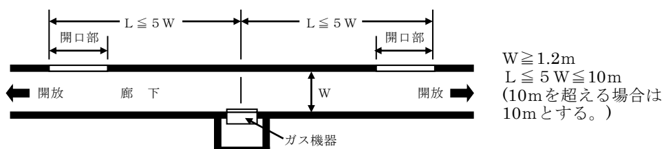
第 12－4 図 開口部の範囲の例
