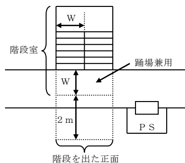
(屋外階段の例)
