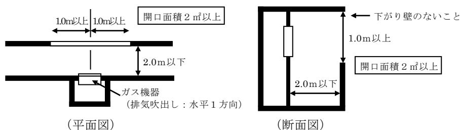
第 12-6 図 前面開口部条件の例
