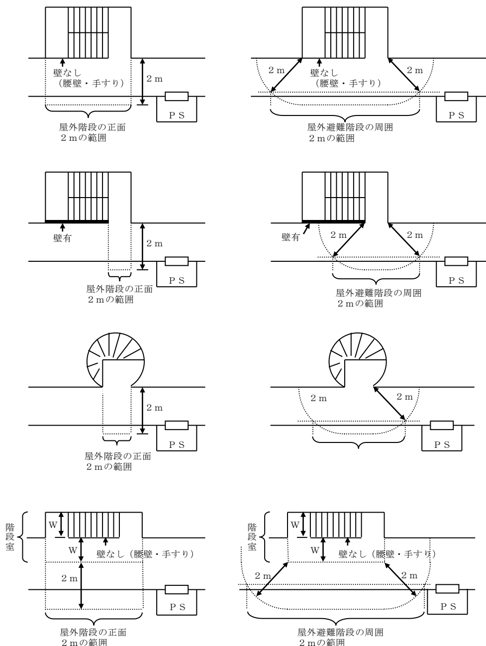
第 12－15 図 屋外階段を出た正面又は屋外避難階段の周囲 2 m を避けた設置例
