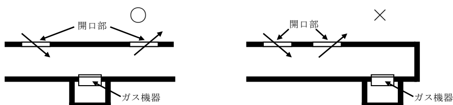
第 12－3 図 廊下等の開放条件の例
