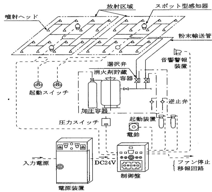
別図第 10-1 粉末消火設備系統図
