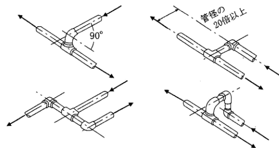
別図第 10-2 粉末消火設備における T 型継手の良い配管方法
