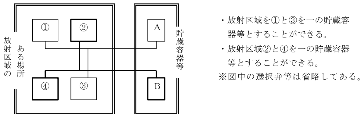
第 10－2 図 並列の放射区域ごとの貯蔵容器等の組合せ例
