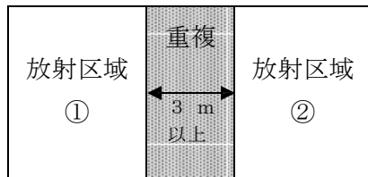
第 10－4 図 2 放射区域のみで 3 m 以上の重複がある場合の消火剤の貯蔵量の例
