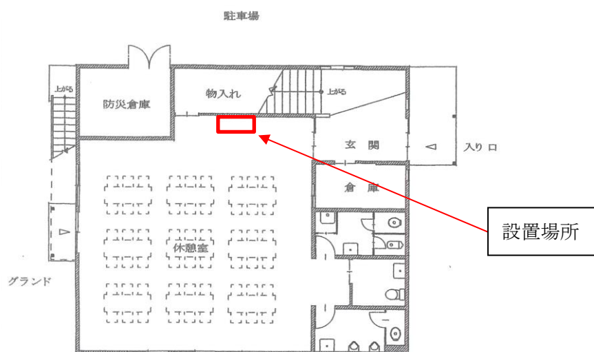
1 階平面図
