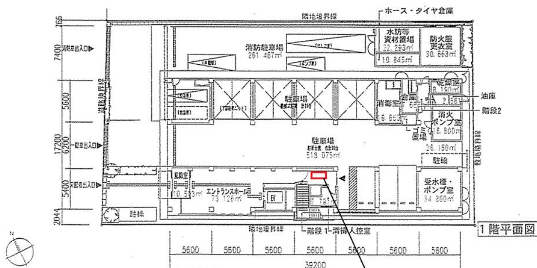
各階平面図
