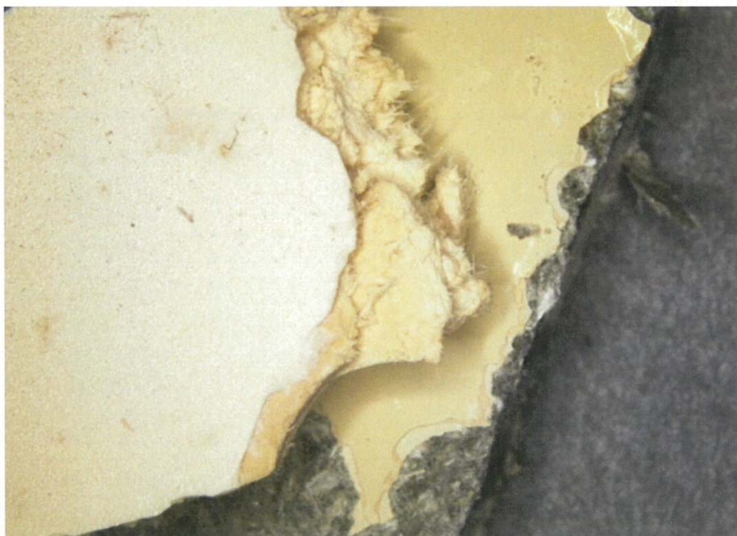
試料表面
