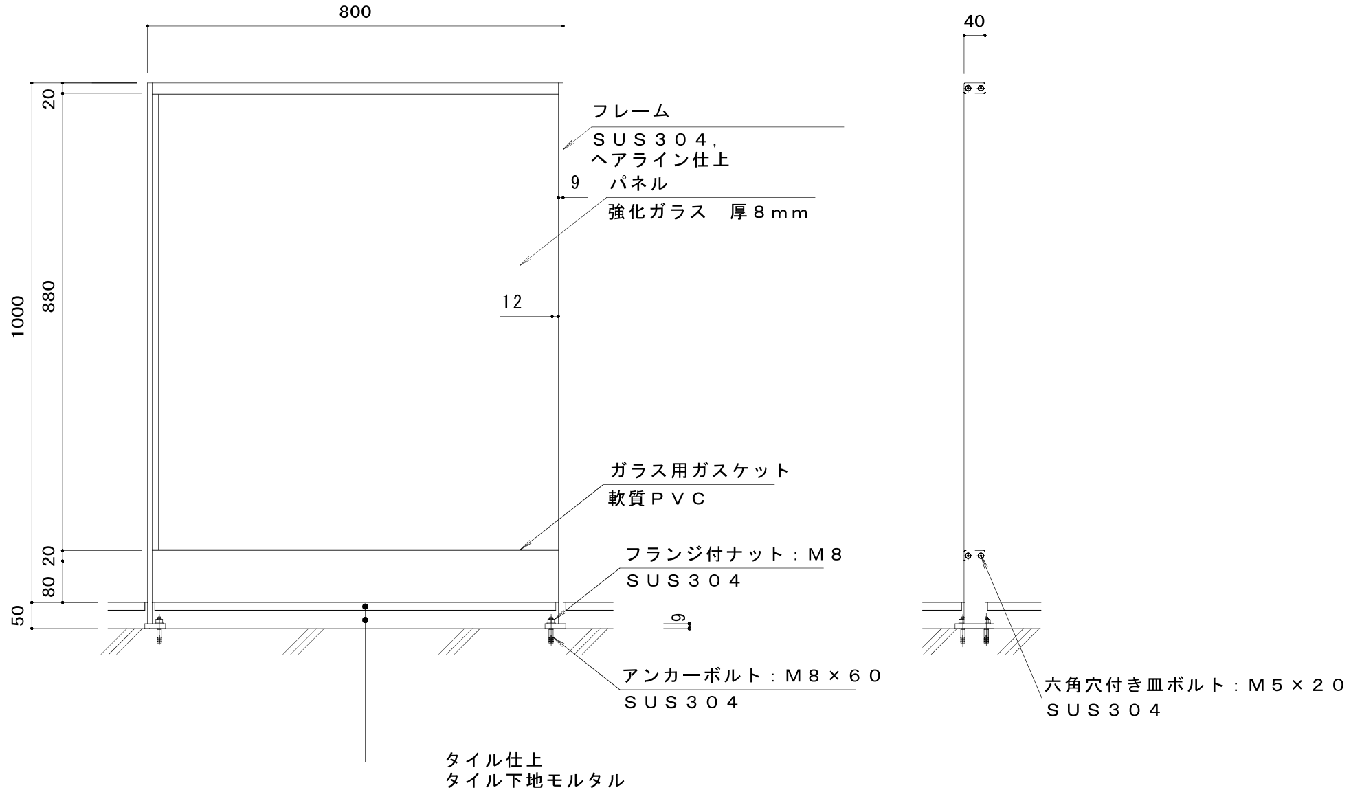
自動ドア防護柵(参考図)
