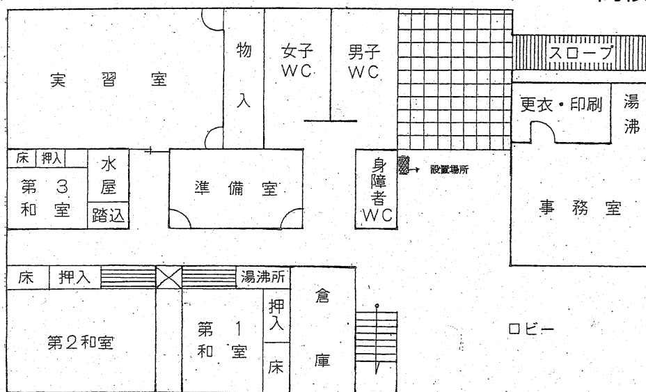
1階 高根公民館 平面図
