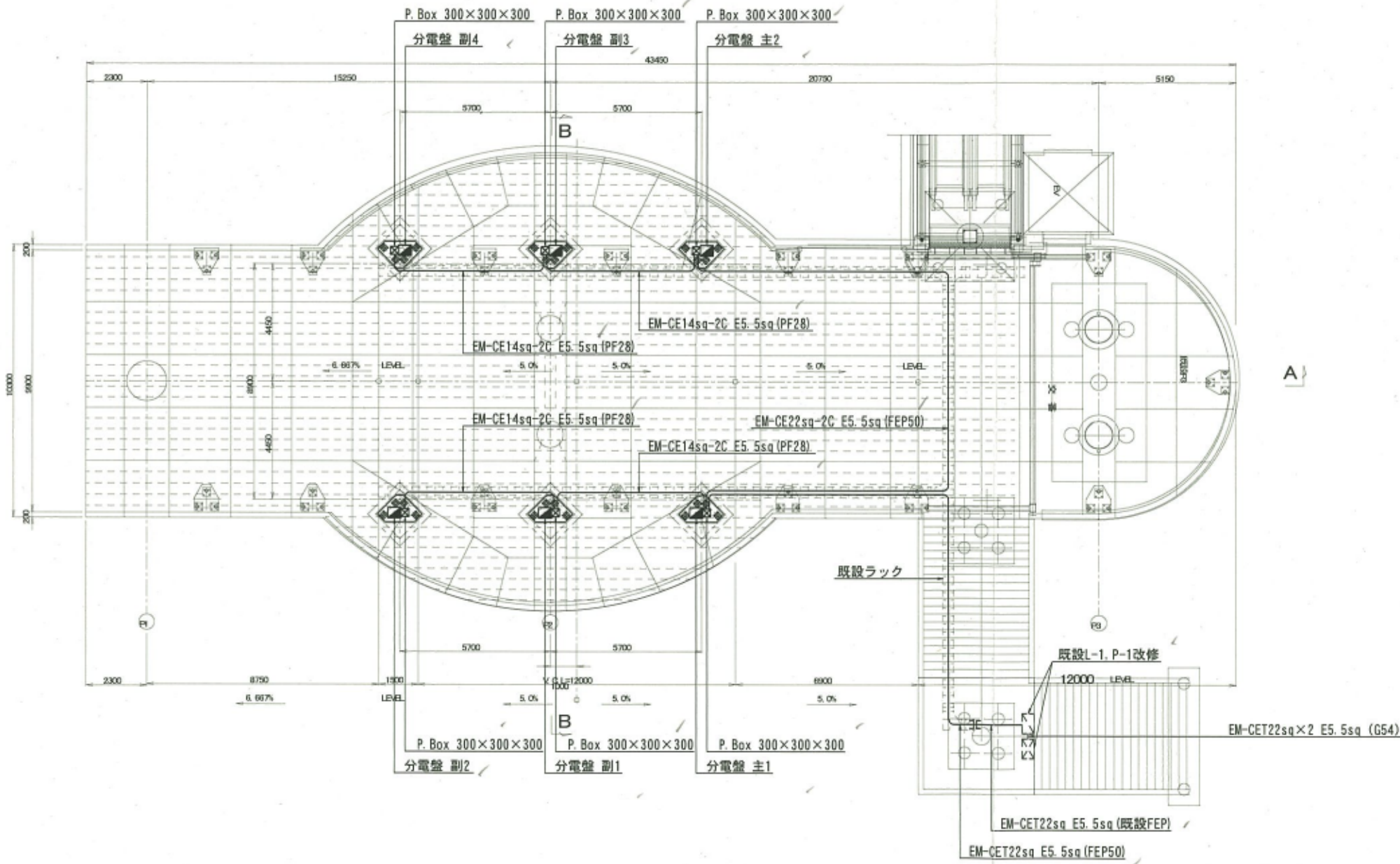
平面図 S=1:200
