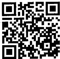
iOS 版
