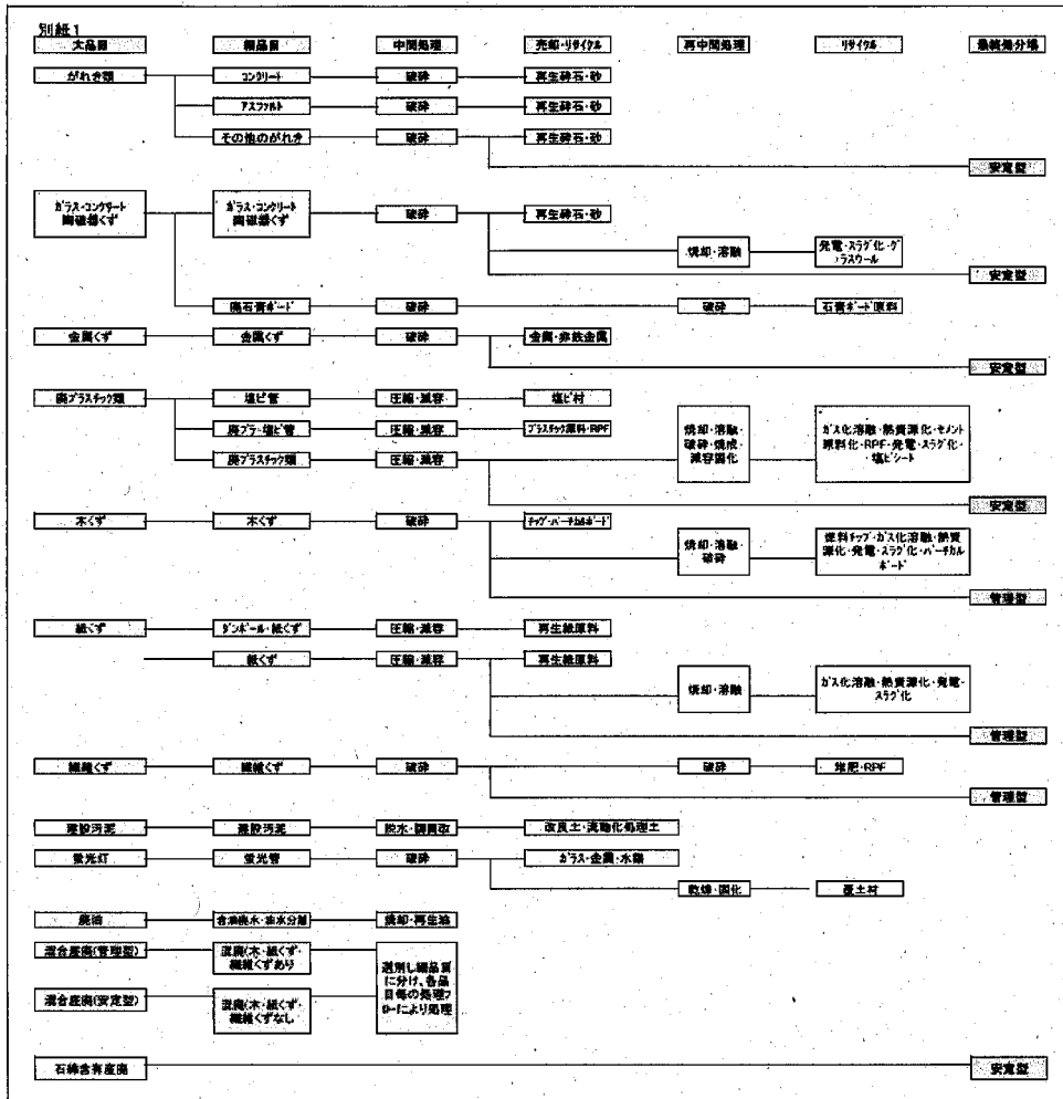
別添 1 処理工程図
