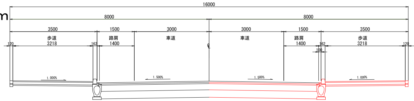
標準横断面図
