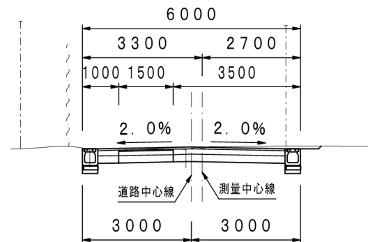
標準断面図
