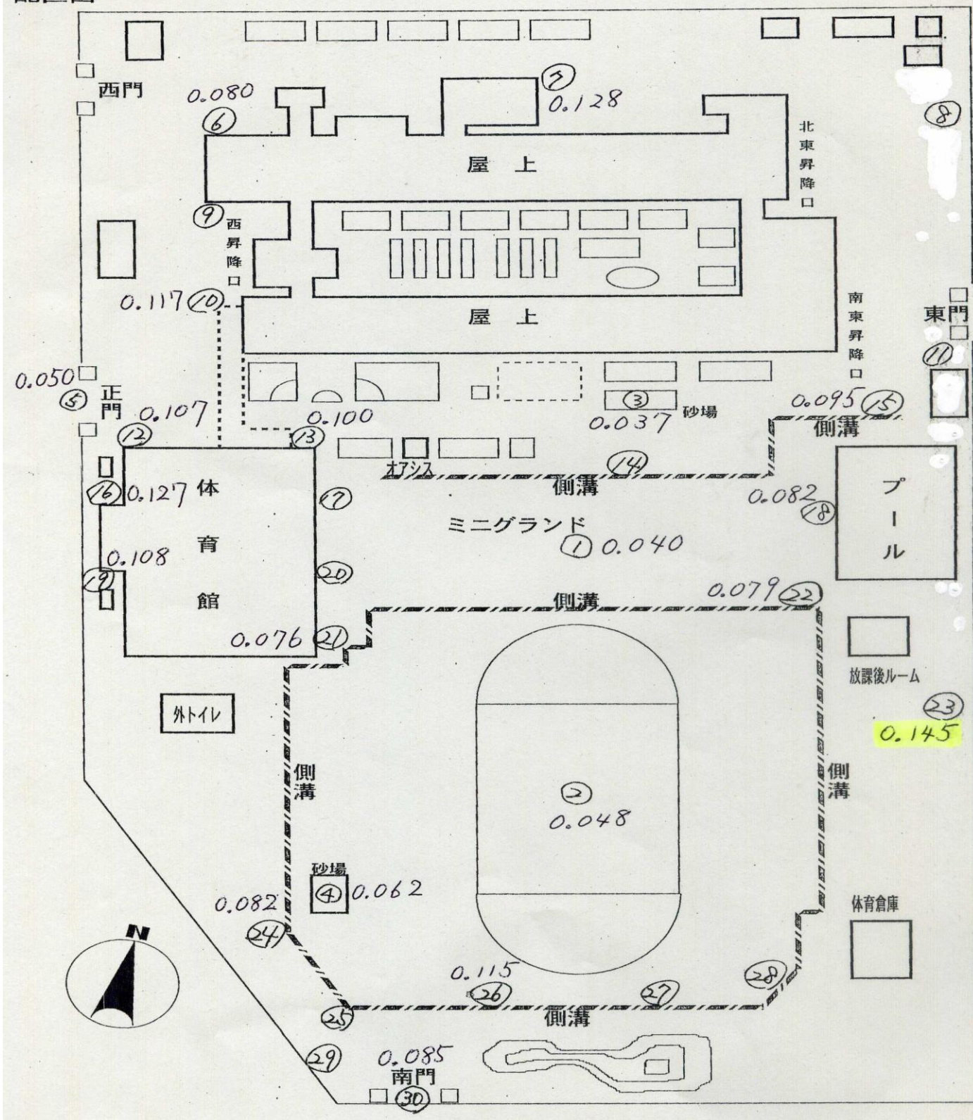
配置図
