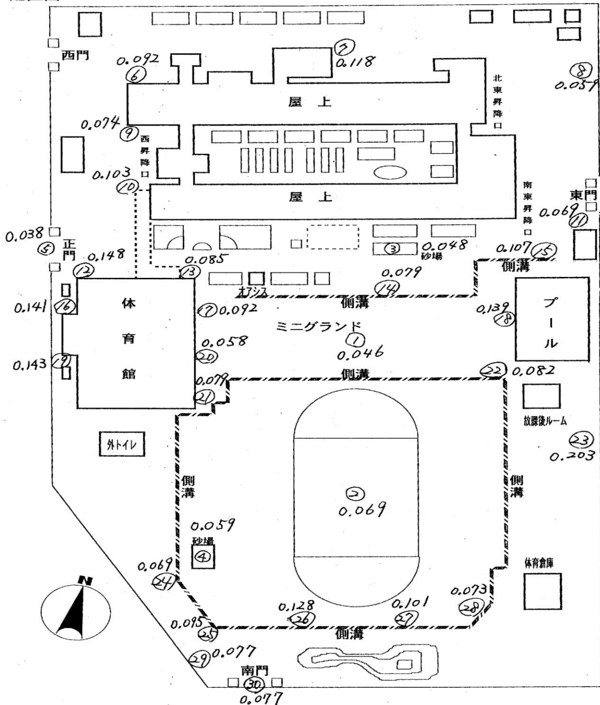
配置図
