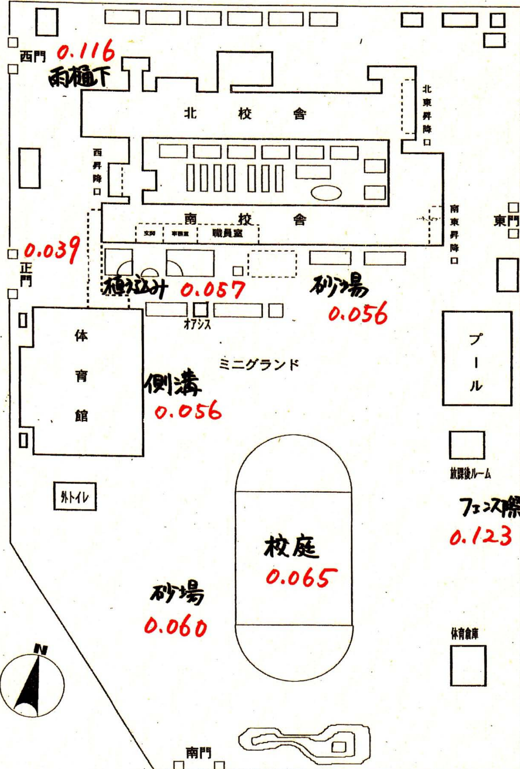
校舎配置図
